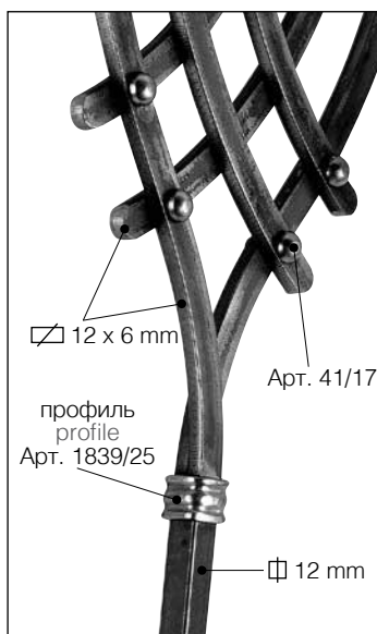
Арт. GD20/5 □ 12 mm H 1000 mm L 180 mm
