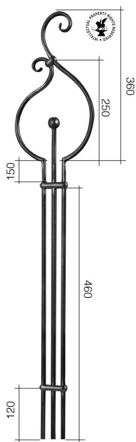
Арт. GD39/1 Ø 12 mm L 200 mm H 1000 mm
