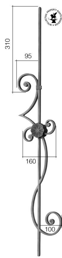
Арт. GD191/1 14 x 8 mm L 180 mm H 1000 mm
