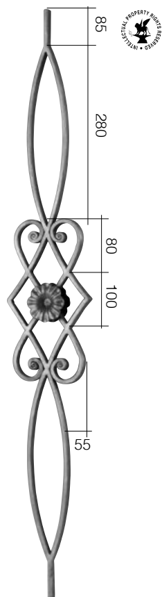
Арт. GD16/1 □ 14 x 8 mm L 160 mm H 1000 mm
