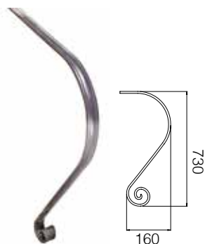
Арт. 114/B/15 for handrail окончание для перил арт. 114/A/3
