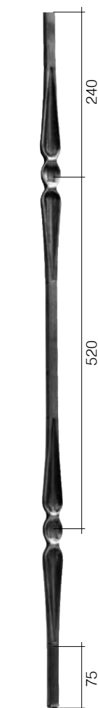
Арт. 1749/3 \Phi 12 x 12 mm L 25 mm H 1000 mm
