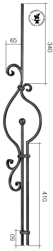
Арт. GD39/3 Ø 12 mm L 190 mm H 1000 mm
