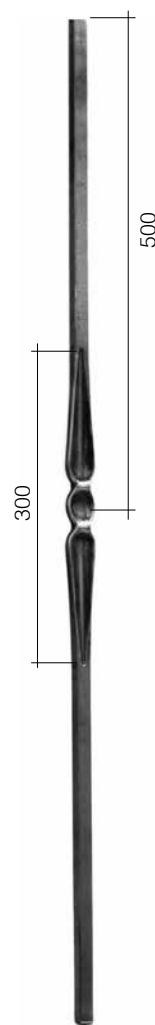
Арт. 1749/1 \Phi 12 x 12 mm L 25 mm H 1000 mm
