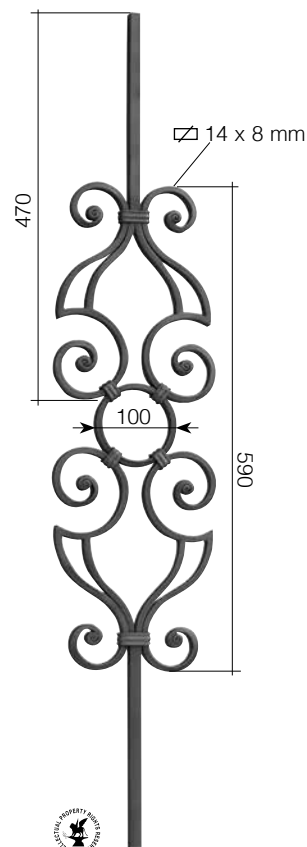
Арт. GD151/1 □ 14 mm L 205 mm H 1000 mm
