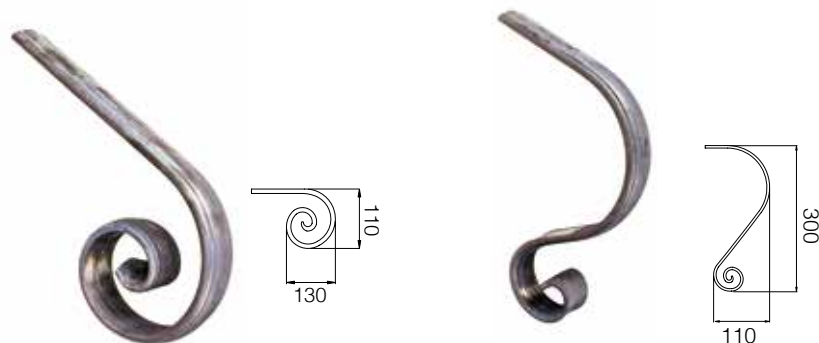
Арт. 116/10 for handrail окончание для перил Арт. 114/5
