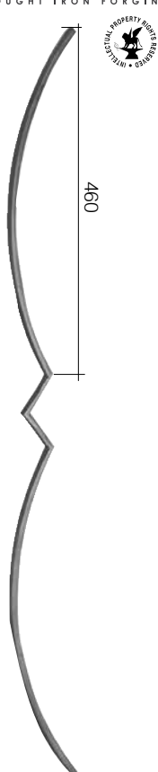
Арт. GD12/1 □ 14 x 8 mm L 95 mm H 1000 mm
